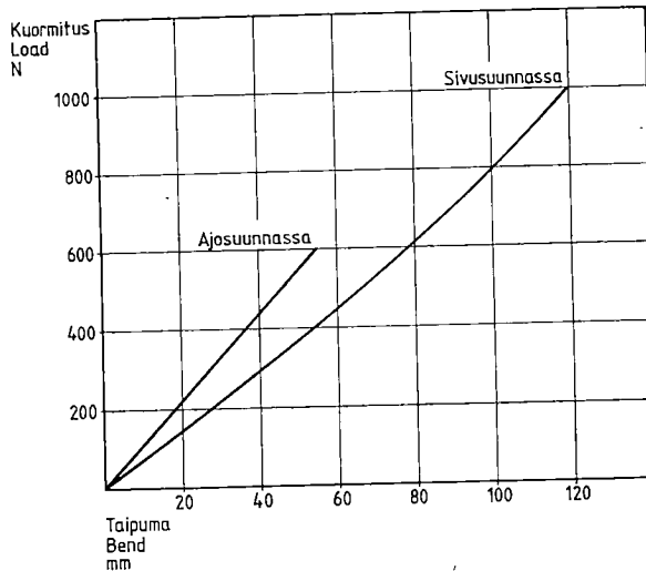
Kuva 1. Piihin taipuma ilman terää Figure 1. Bending of tine without shovel
