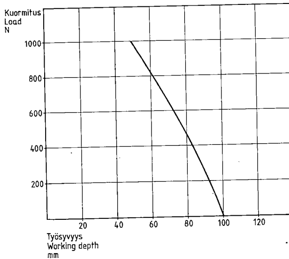
Kuva 2. Piihin työsyvyyden muuttuminen kärjestä mitattuna Figure 2. Variation of working depth measured at the point
