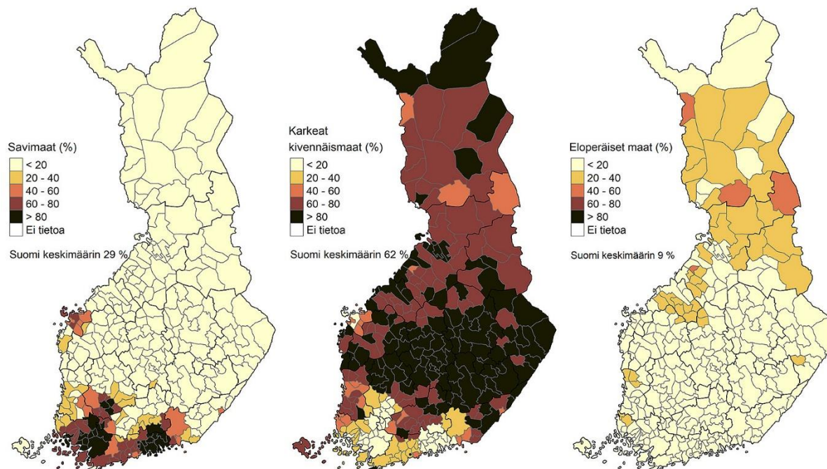
Kuva 3. Savimaiden, karkeiden kivennäismaiden ja eloperäisten maiden osuus (%) kunnan pelto- maista. Kuntien aluerajat on merkitty harmaalla ja ELY-keskusten mustalla viivalla. Ahvenan- maata käsitellään yhtenä kokonaisuutena.
