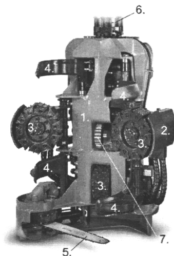
Рисунок 2.11. Харвестерная головка фирмы «Понссе». 1 – рама; 2 – захватные рычаги; 3 – подающие вальцы; 4 – сучкорезные ножи; 5 – пила; 6 – поворотный ротор; 7 – механизм измерения длины. (Фотография: АО «Понссе»)
