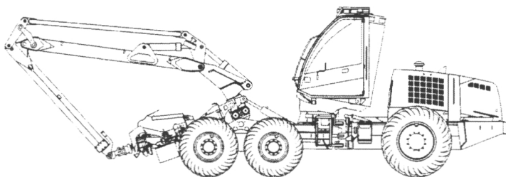
Рисунок 2.10. Компонировочное решение харвестера с задним моторным модулем (Timberjack 1270). (Рисунок: АО «Тимберджек»)
