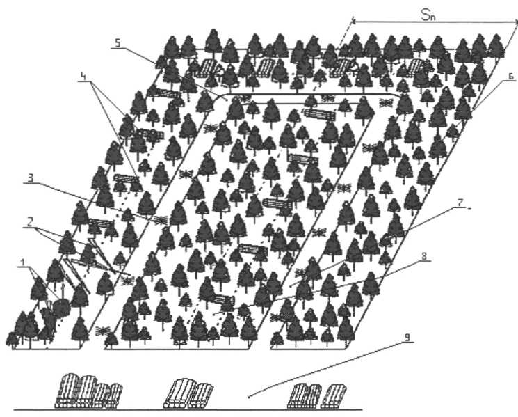
Рисунок 2.25. Схема разработки ленты, удаленной от волока: 1 – поваленные деревья; 2 – сортименты; 3 – порубочные остатки; 4 – пачки сортиментов; 5 – разворотное кольцо; 6 – растущий лес; 7 – пасечный волок; 8 – лента, удаленная от волока; 9 – лесопогрузочный пункт; S_n – ширина пасеки.
