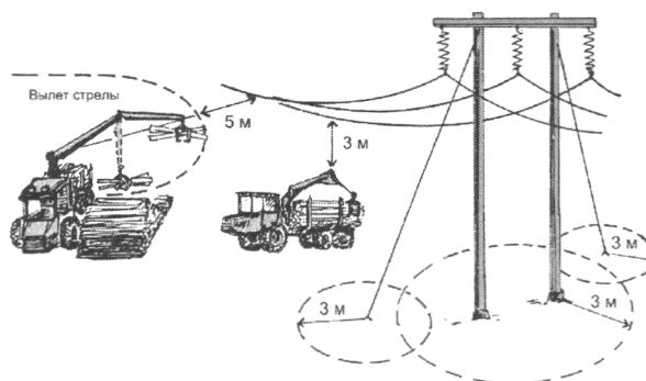
Рисунок 4.2. Схема зон безопасности (финский пример). (Рисунок: АО «Метсätэхo»)
