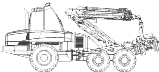
Рисунок 2.9. Компонировочное решение харвестера с передним моторным модулем (Ponsse Ergo). (Рисунок: АО «Понссе»)
