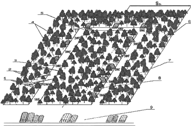
Рисунок 2.24. Схема разработки ленты, примыкающей к волоку: 1 – поваленные деревья; 2 – сортименты; 3 – порубочные остатки; 4 – пачки сортиментов; 5 – разворотное кольцо; 6 – растущий лес; 7 – пасечный волок; 8 – лента, примыкающая к волоку; 9 – лесопогрузочный пункт; S_n – ширина пасеки.
