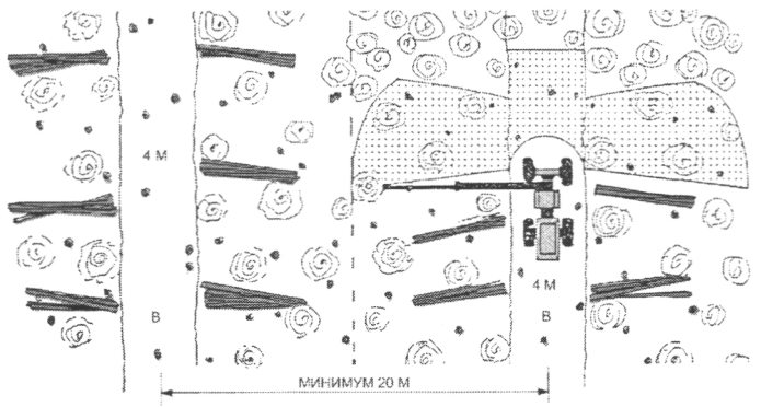
Рисунок 2.27. Типовая схема работы харвестера при расстоянии между волоками 20 м. (Рисунок: АО «Метсятэхо»)
