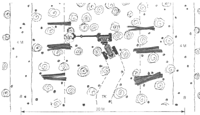
Рисунок 2.28. Допустимая схема работы харвестера при расстоянии между волоками более 20 м. (Рисунок: АО «Метсятэхо»)
