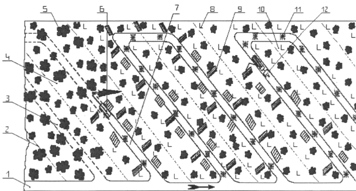
Рисунок 2.26. Типовая технологическая схема разработки лесосеки с использованием харвестера и форвардера: 1 – магистральный волок; 2 – граница посеки; 3 – размеченный волок (до рубки); 4 – полупосека до рубки; 5 – растущее дерево; 6 – харвестер; 7 – прорубленный волок; 8 – пень; 9 – пачка сортиментов; 10 – полупосека после рубки; 11 – порубочные остатки; 12 – форвардер; ➔ – направление перевозки сортиментов на лесопогрузочный пункт.
