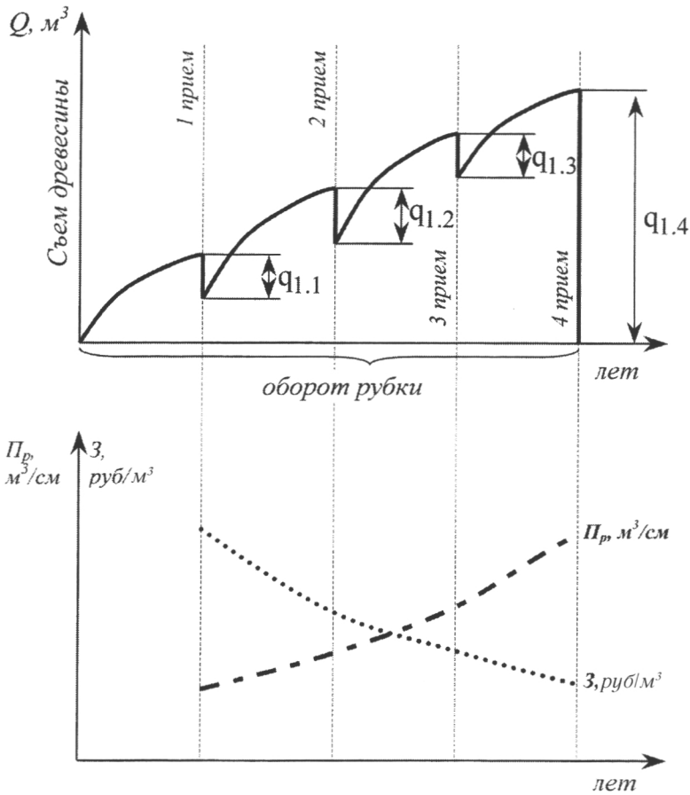
Рисунок 3.8. Графическое представление критериев эффективности четырехприемной рубки: Q – срез древесины, м^3 ; Пр – производительность, м^3/смена ; З – затраты, руб/м^3 .
