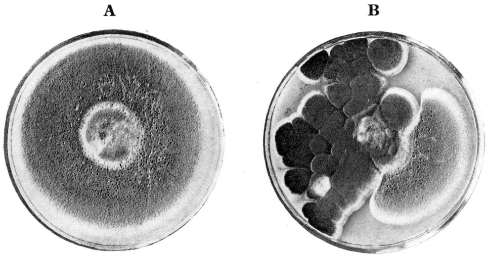
Abb. 6. Gloeosporium agaves auf Haferschleim-Agar (Orig.). Kuva 6. Gloeosporium agaves kauraliemiagarilla.
