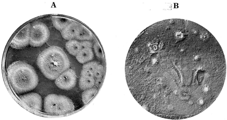
Abb. 7. A = Gloeosporium (Colletotrichum) agaves . Kuva 7 B = Glomerella cingulata (Orig.).
