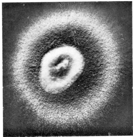
Abb. 5. Gloeosporium agaves -Kolonie auf Haferschleim-Agar. Vergr. 10 × (Orig.).*)
