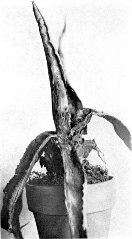
Abb. 1. Colletotrichum Agaves . Durch den Pilz verursachte Flecken an den Blättern von Agave americana (Orig.).
