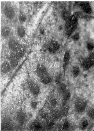
Abb. 3. Konidienhaufen an der Oberfläche eines Blattes (Orig.).
