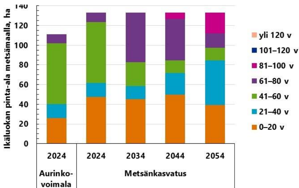
Kuva 5. Puuston ikäluokittaiset pinta-alat (ha) metsämaalla lasketuissa skenaarioissa 2024–2054 Kyyrönsuon suunnitelma-alueella. Metsänkasvatus -skenaariossa metsämaan ala lisään-tyy 26 hehtaarilla entistä turvetuotantoaluetta, joka metsitetään vuonna 2024.
