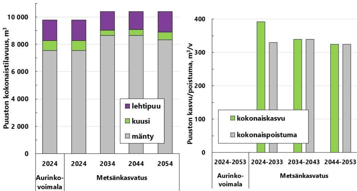
Kuva 3. Runkopuun kokonaistilavuudet (m 3 ) puulajeittain (vasemmalla) sekä vuotuiset kokonaiskasvut ja -poistumat (m 3 /vuosi) (oikealla) lasketuissa skenaarioissa ajanjaksolla 2024–2054 Paiholan suunnitelma-alueella.
