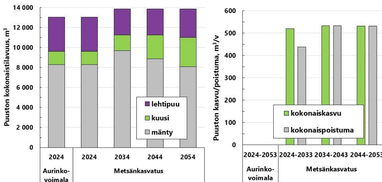
Kuva 6. Runkopuun kokonaistilavuudet (m 3 ) puulajeittain (vasemmalla) sekä vuotuiset kokonaiskasvut ja -poistumat (m 3 /vuosi) (oikealla) lasketuissa skenaarioissa ajanjaksolla 2024–2054 Kyyrönsuon suunnitelma-alueella.
