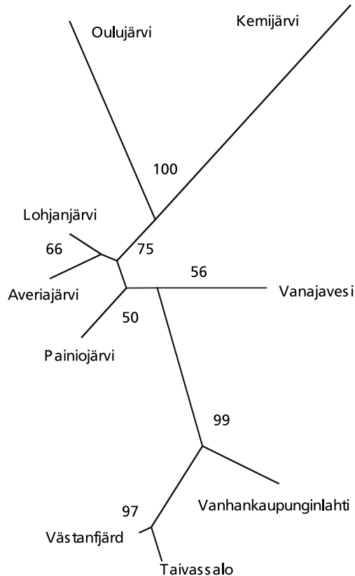
Kuva 3. Juureton dendrogrammi tutkituista kuhapopulaatioista. Puiden haarojen sijainnin todennäköisyys on ilmaistu prosentteina. Populaatioita yhdistävien viivojen pituudet kuvastavat niiden välisiä perinnöllisiä etäisyyksiä.
