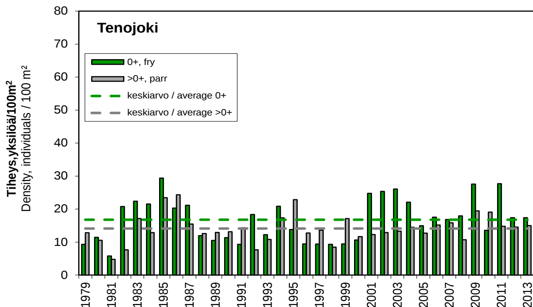
Kuva 11. Kesänvanhojen (0+) ja vanhempien (>0+) lohenpoikasten vuosittaiset keskitiheydet Tenon pääuoman koekalastusalueilla (n=22) vuosina 1979–2013. Katkoviivoilla on merkitty pitkän aikavälin (1979–2013) ikäryhmäkohtaiset keskitiheydet. Kaikki tiheydet perustuvat yhden sähkökalastuskerran tuloksiin.
