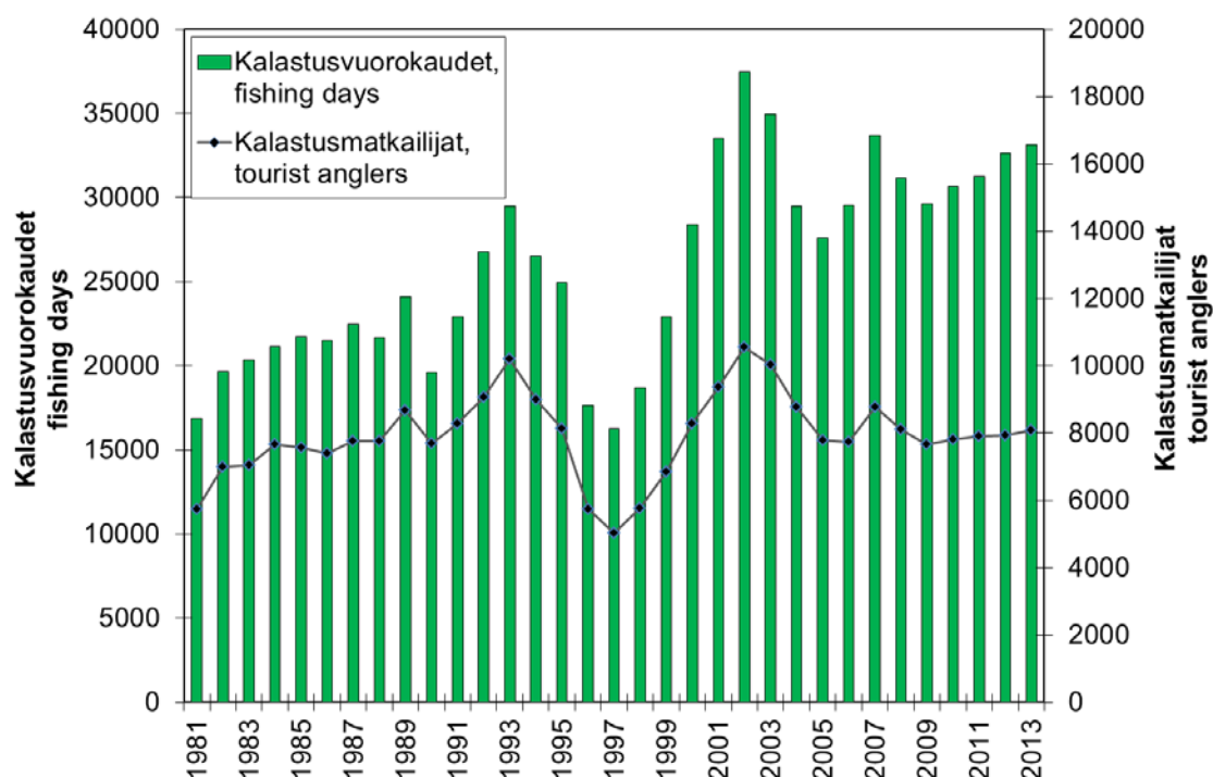
Kuva 3. Kalastusmatkailijat ja kalastusvuorokaudet Suomessa Teno-Inarijoen rajajokialueella v.1981–2013.
