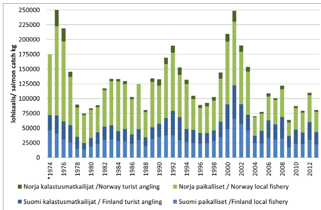
Kuva 5. Paikkakuntalaisten ja kalastusmatkailijoiden lohisaalis Tenojoen vesistöalueelta Suomessa ja Norjassa v. 1974–2013. *Vuosille 1974 ja 1987 Norjassa ei arvioitu erikseen kalastusmatkailijoiden lohisaalista.
