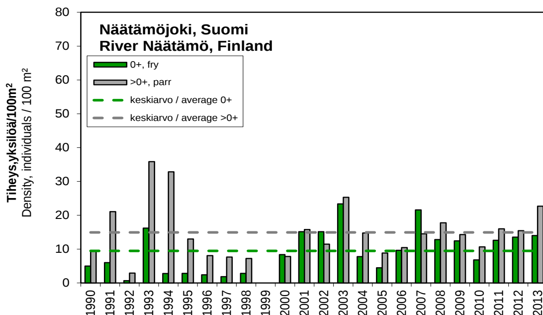
Kuva 15. Kesänvanhojen (0+) ja vanhempien (>0+) lohenpoikasten vuosittaiset keskitiheydet (kpl/100 m 2 ) Näättäjäjoen Suomen puoleisilla koekalastusalueilla vuosina 1990–2013. Katkoviivoilla on merkitty pitkän aikavälin (1990–2013) ikäryhmäkohtaiset keskitiheydet. Kaikki tiheydet perustuvat yhden sähkökalastuskerran tuloksiin.
