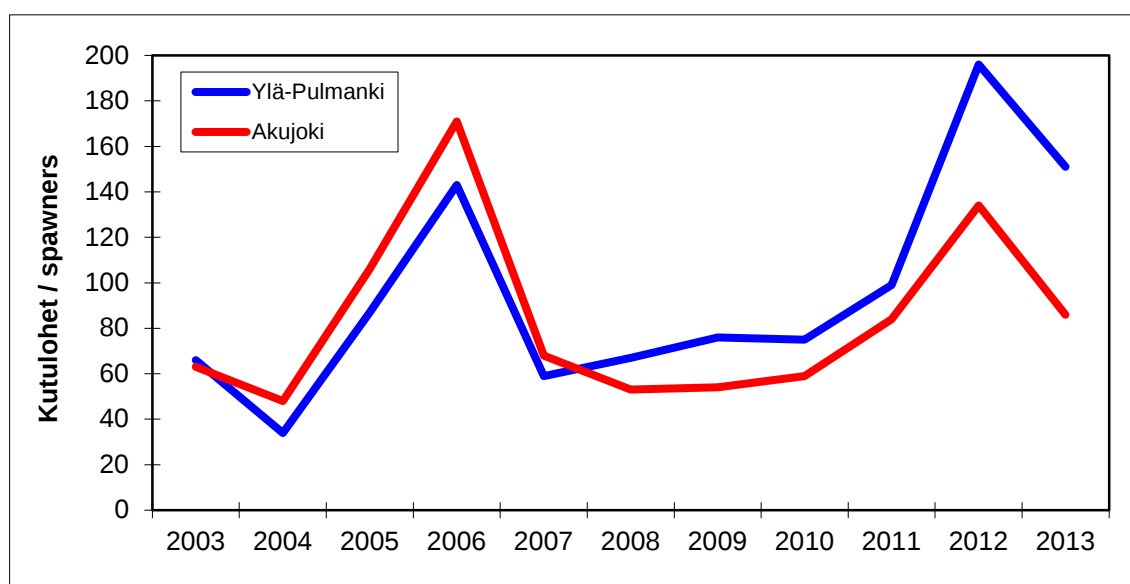
Kuva 20. Ylä-Pulmanki- ja Akujoella pintasukelluslaskennoissa havaittujen kutulohien määrät vuosina 2003–2013.
