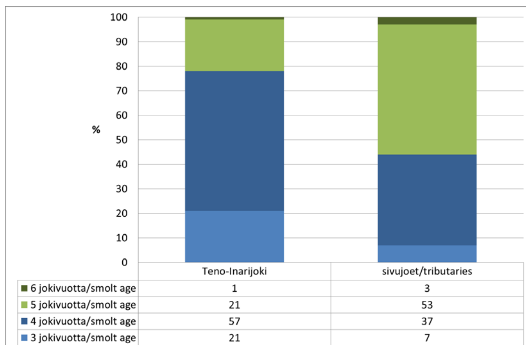
Kuva 8. Teno-Inarijoen pääuoman ja Tenojoen Suomen puolen merkittävimpien sivujokien (Pulmankijoki, Vetsijoki ja Utsjoki) saalislohiin joki-ikäjakauma (%) suomenäyteaineistossa v. 2013.
