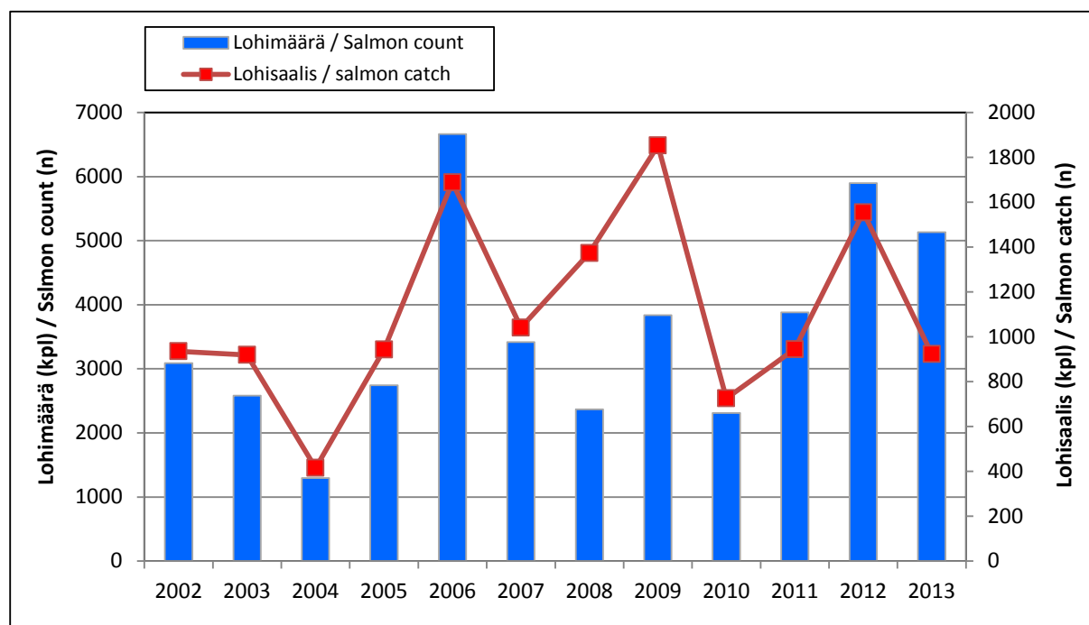
Kuva 17. Utsjoen videoseurannassa havaitut nousulohien määrät (kpl) ja arvioitu saalislohiemäärä (kpl) Utsjoen vesistöalueelta vuosina 2002–2013. Vuosien 2005 ja 2011 videoaineistot ovat osin puutteellisia, koska kamerat saatiin kyseisinä vuosina asennettua tavanomaisista myöhemmin.
