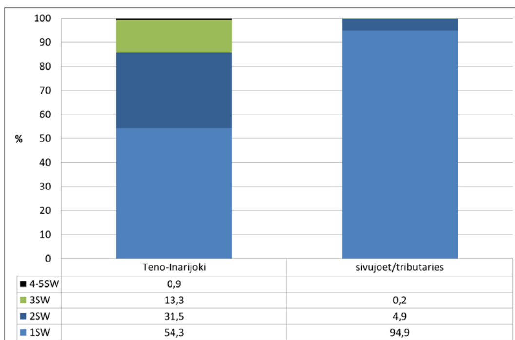
Kuva 9. Teno-Inarijoen pääuoman ja Tenojoen Suomen puolen merkittävimpien sivujokien (Pulmankijoki, Vetsijoki, Utsjoki) saalislohien meri-ikäjakauma (%) suomenäyteaineistossa v. 2013.
