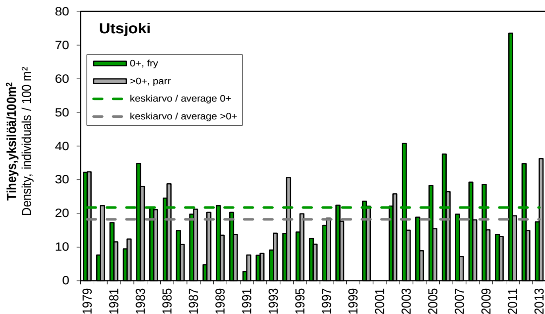
Kuva 12. Kesänvanhojen (0+) ja vanhempien (>0+) lohenpoikasten vuosittaiset keskitiheydet Utsjoen koekalastusalueilla vuosina 1979–2013. Katkoviivoilla on merkitty pitkän aikavälin (1979–2013) ikäryhmäkohtaiset keskitiheydet. Kaikki tiheydet perustuvat yhden sähkökalastuskerran tuloksiin.
