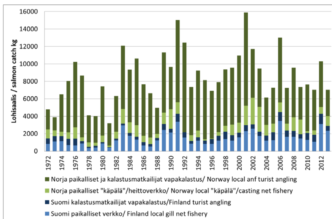
Kuva 6. Paikkakuntalaisten ja kalastusmatkailijoiden lohisaalis (kg) Näättämojoesta Suomessa ja Norjassa v. 1972–2013.
