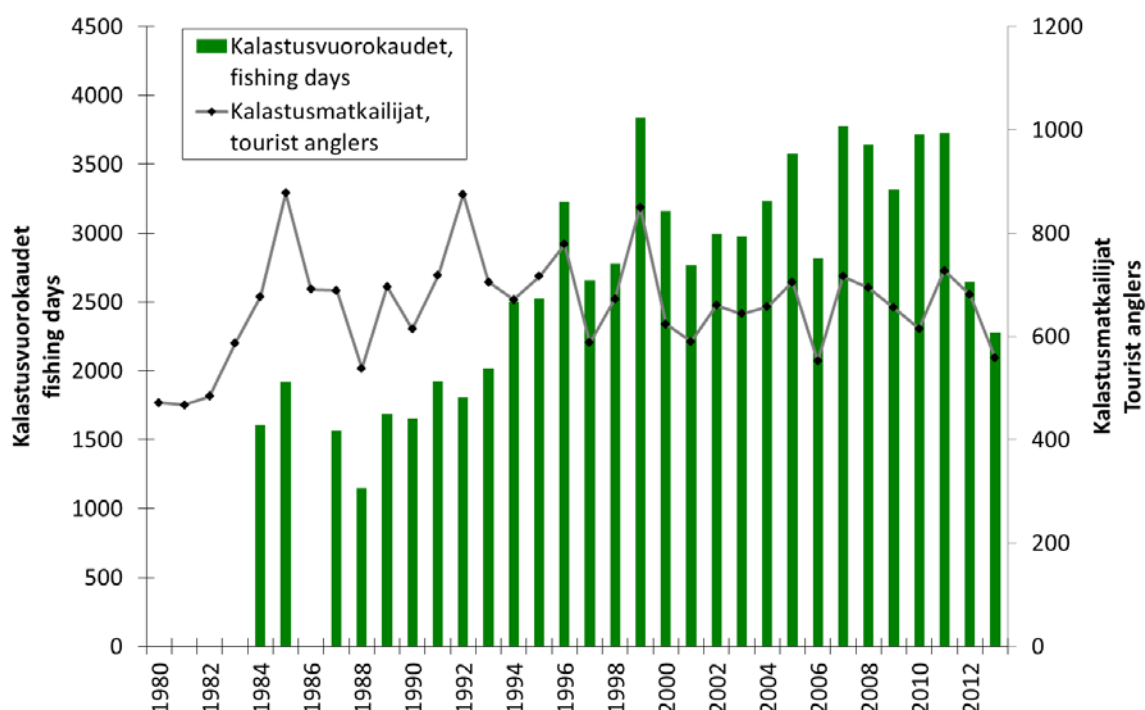
Kuva 4. Näättäjäjoen kalastusmatkailijoiden ja kalastusvuorokausien määrät Suomen puolella v. 1980–2013. Vuosina 1994–2011 myytiin edullisia viikkolupia (7 vrk), joiden myynti lopetettiin v. 2012.
