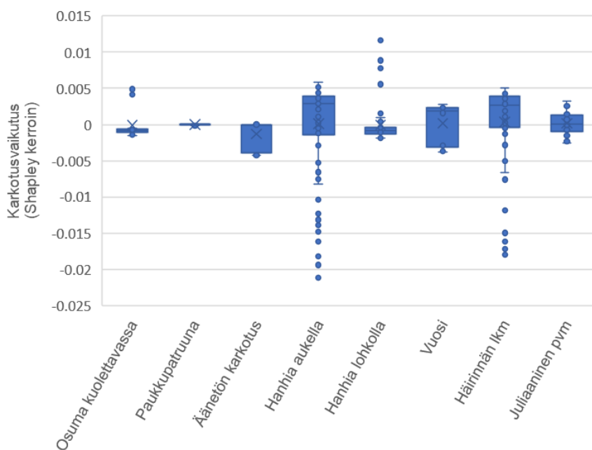
Kuva 20. Käsittelyjen (kuolettava ampuminen, paukkupatruuna ja äänetön karkotus) karkotusvaikutus (Shapley kerroin; y-akseli: + = hanhiparvi poistuu peltoaukealta, - = hanhiparvi ei poistu peltoaukealta) per näyte (aineiston rivi), sekä muiden mallissa mukana olleiden tekijöiden vaikutus karkotukseen.
