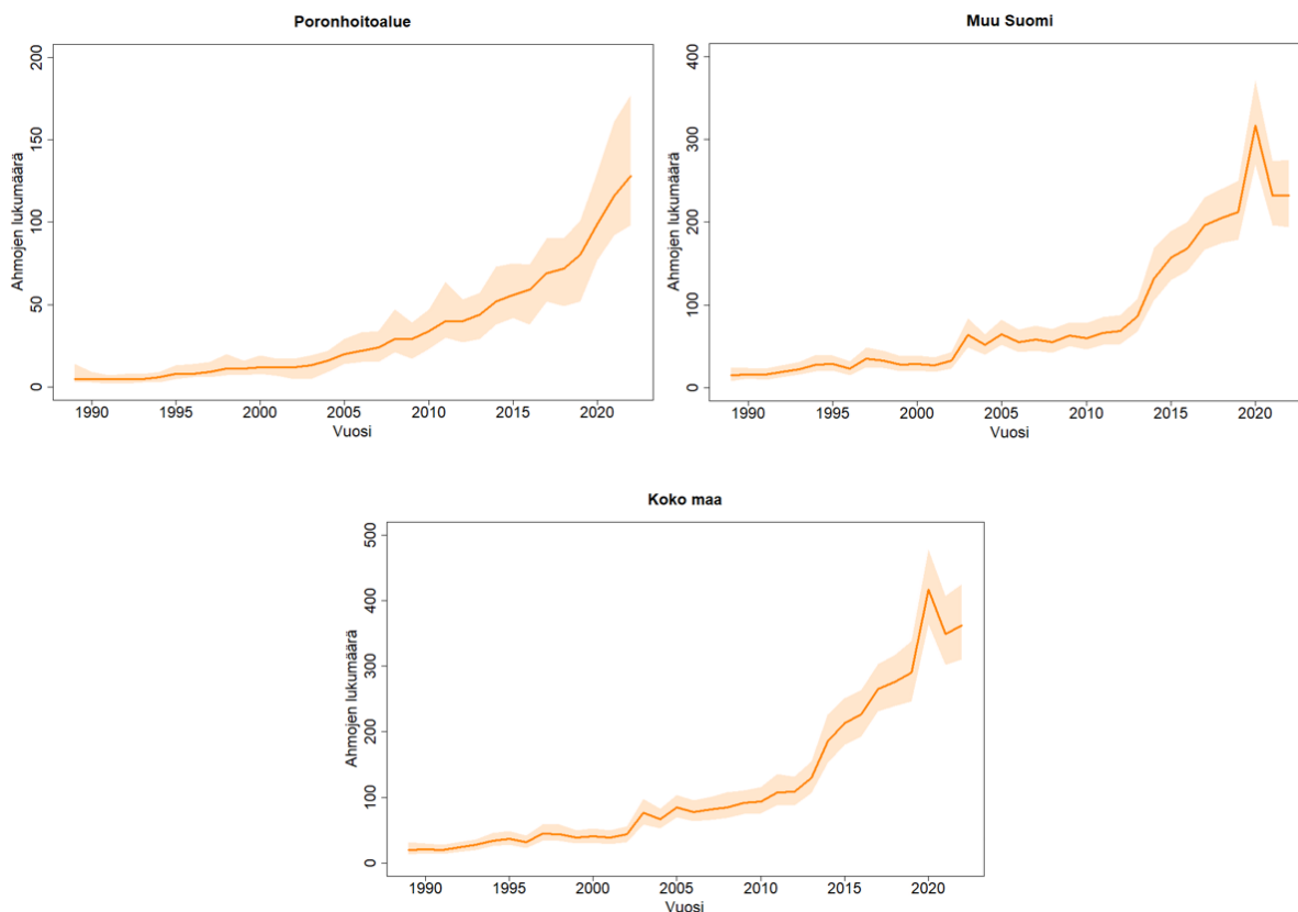
Kuva 1. Ahmojen todennäköisin yksilömäärä ja 95 %:n todennäköisyysväli riistakolmioaineis- tossa vuosina 1989–2022. Todennäköinen yksilömäärä laskettuna poronhoitoalueelle ja muulle Suomelle sekä yhdistettynä koko Suomen alueelle.
