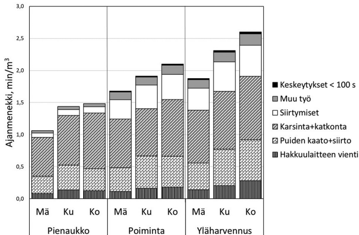
Kuva 4. Ajanmenekki ainespuukuutiometriä kohden ( \text{min}/\text{m}^3 ) työvaiheittain.
