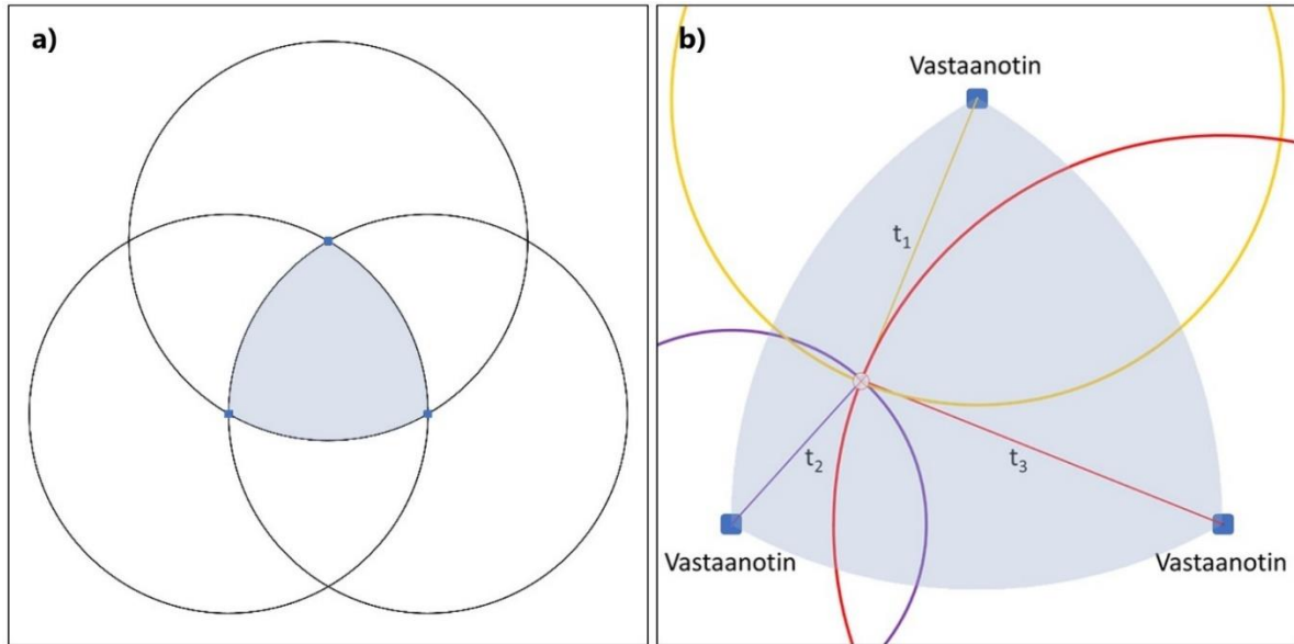
Kuva 6. Havainnekuva kolmiomittauksen periaatteesta. a) Vastaanottimien (■) kuuluualue (musta ympyrä) rajaa mittatarkkuuden kannalta parhaan alueen (harmaa). b) t_1 , t_2 ja t_3 kuvaavat aikaa/matkaa, joka signaalilta kuluu lähettimeltä (⊗) vastaanottimelle.
