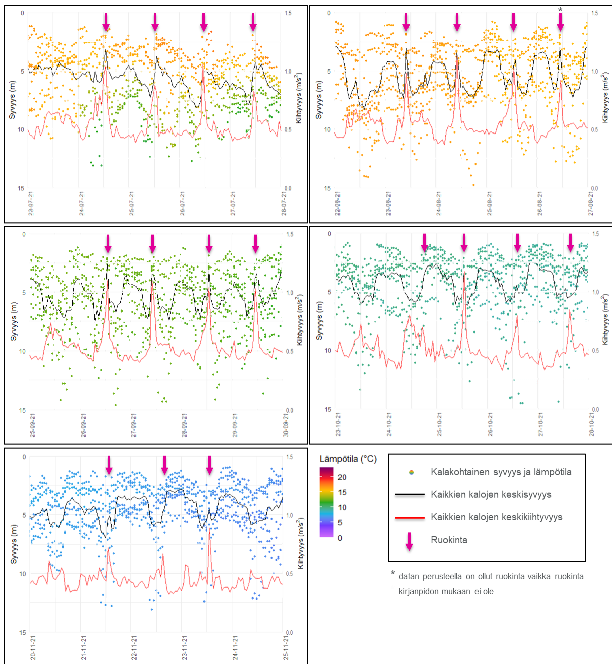
Kuva 32. Kalojen syvyys, lämpötila ja kiihtyvyys tuntikohtaisina keskiarvoina 5 vrk ajan eri kuu- kausina, kun kaloja on voitu ruokkia yhtäjaksoisesti 3–4 vuorokautena tarkastelujakson aikana.
