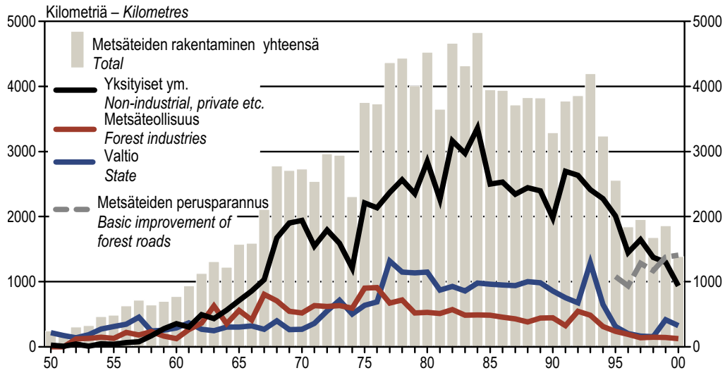
Kuva 3.9 Metsäteiden rakentaminen ja perusparannus 1950–2000 Figure 3.9 Construction and basic improvement of forest roads 1950–2000
