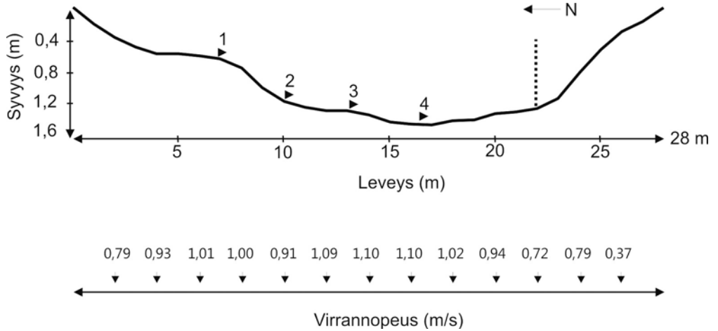
Kuva 11. Luttojoen videoseurantapaikan jokiuoman poikkileikkausprofiili ja kameroiden 1–4 sijoituskohdat (yläkuva) sekä jokiuoman pintavirranopeudet (10 cm pinnan alta) mitattuna kahden metrin välein (alakuva). Pystykatkoviiva kuvaa kameran numero neljä maksimaalista kuvausetäisyyttä.
