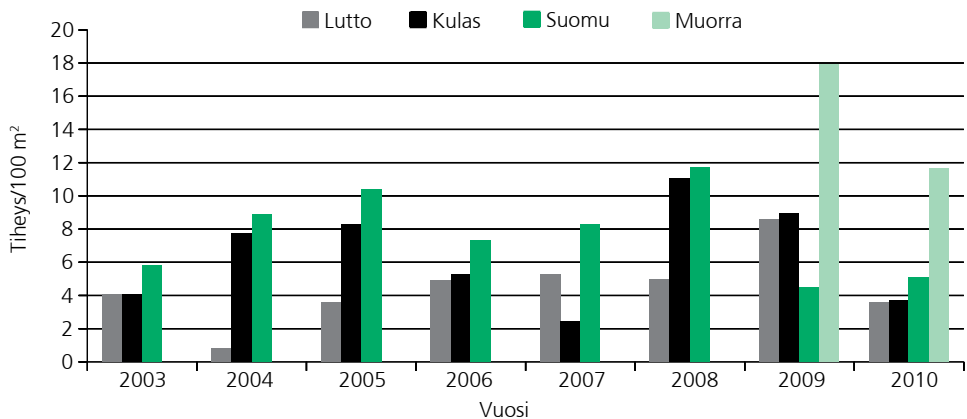
Kuva 3. Luttojen pääuoman (8 koeluetta), Kulasjoen (4 koeluetta), Suomujen (3 koeluetta) ja Muorravaarakkajoen (16 koeluetta) kesänvanhojen (0+) taimenenpoikasten keskitiheys (kpl/100 m 2 ) vuosina 2003–2010 yhden kalastuskerran perusteella.
