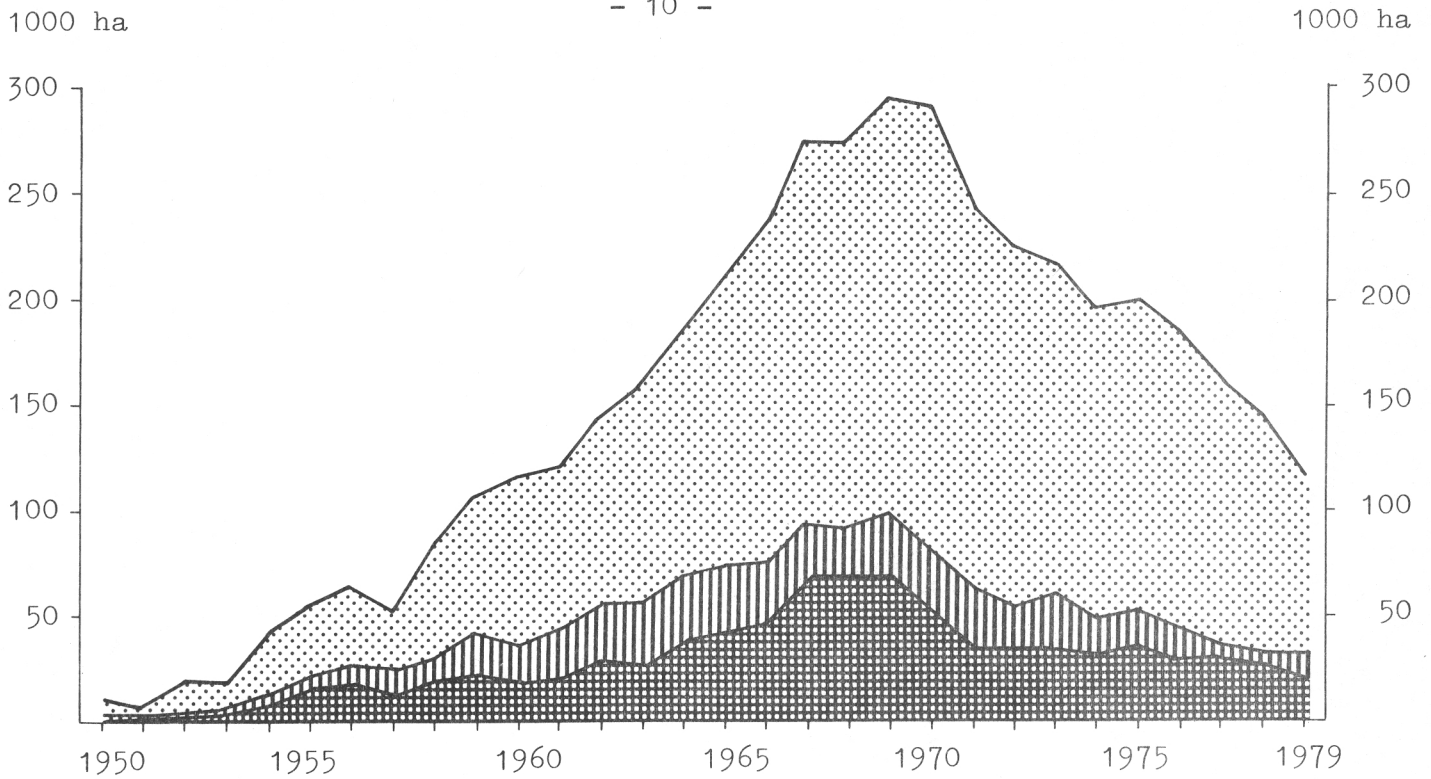
Kuva 4. Metsäojituksen kuivuva ala vuosina 1950-79 metsänomistajaryhmittäin
