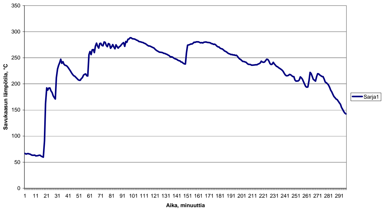
Kuva 11. Savukaasun lämpötila kokeen aikana kun polttoaineena oli olki.
