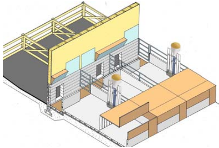
Havainnekuva luomulihasikalan karsinajärjestelyistä ja ulkoilualueesta.
