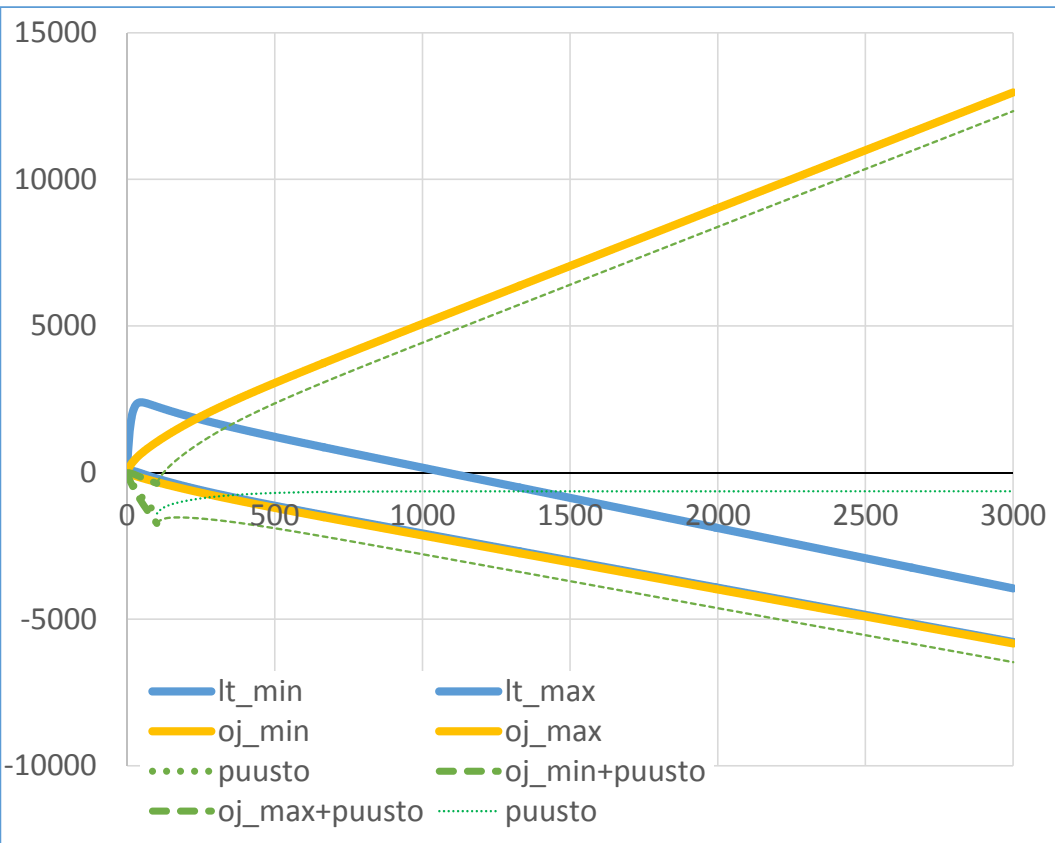
Säteilypakote, \mu\text{W}/\text{m}^2
