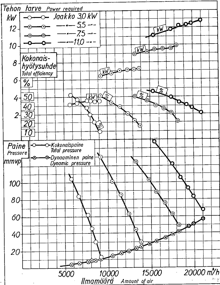
Piirros 1. Jaakko-puhaltimien koetustuloksia. Esitetyt hyötysuhteet ovat puhaltimen ja moottorin yhteisiä kokonaishyötysuhteita.
