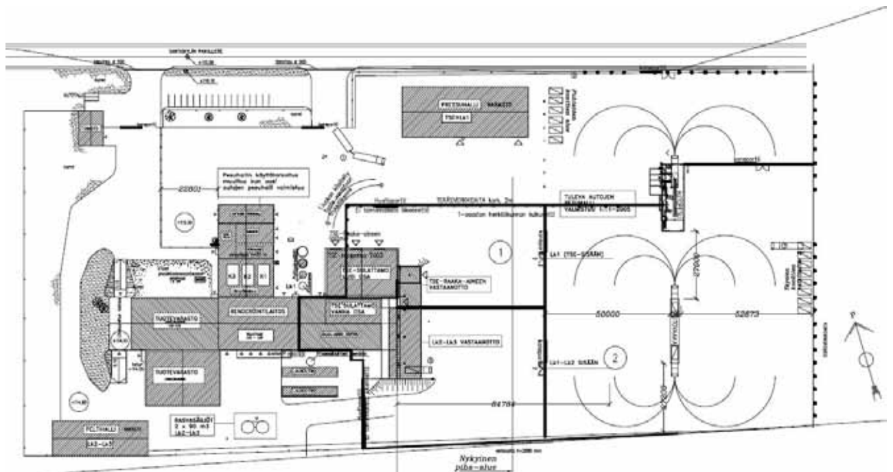
Kuva 4. Honkajoki Oy:n laitosalue, prosessien sijainti.
